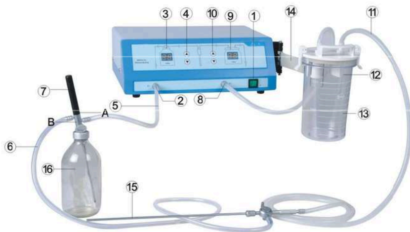
整机示意图
